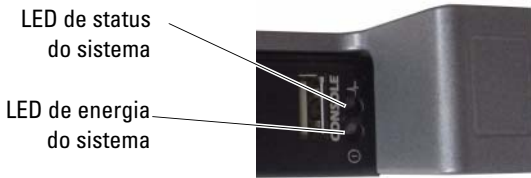
Figura 1-2. LEDs do painel frontal
